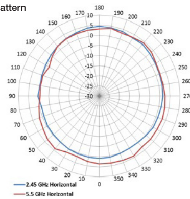
H-Plane Pattern
