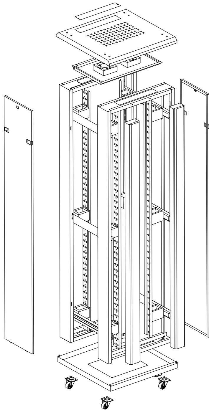
Metalldörr
