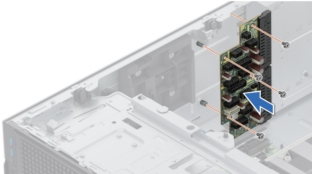
Figure 194. Installation de la carte intercalaire d'alimentation
