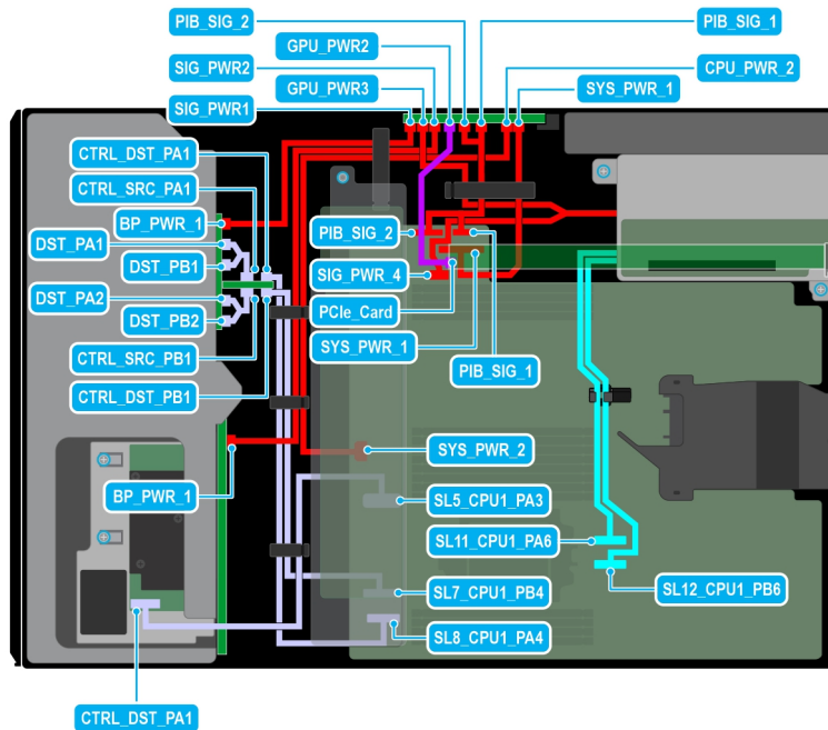
Figure 56. Configuration 18 : 8 disques de 3,5 pouces (SAS/SATA) + 8 disques de 2,5 pouces (NVMe RAID fPERC12) + 1 processeur graphique sur le processeur 1
