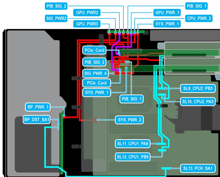
Figure 40. Configuration 2 : 8 disques de 3,5 pouces (Chipset SATA) + 2 processeurs graphiques sur le processeur 2
