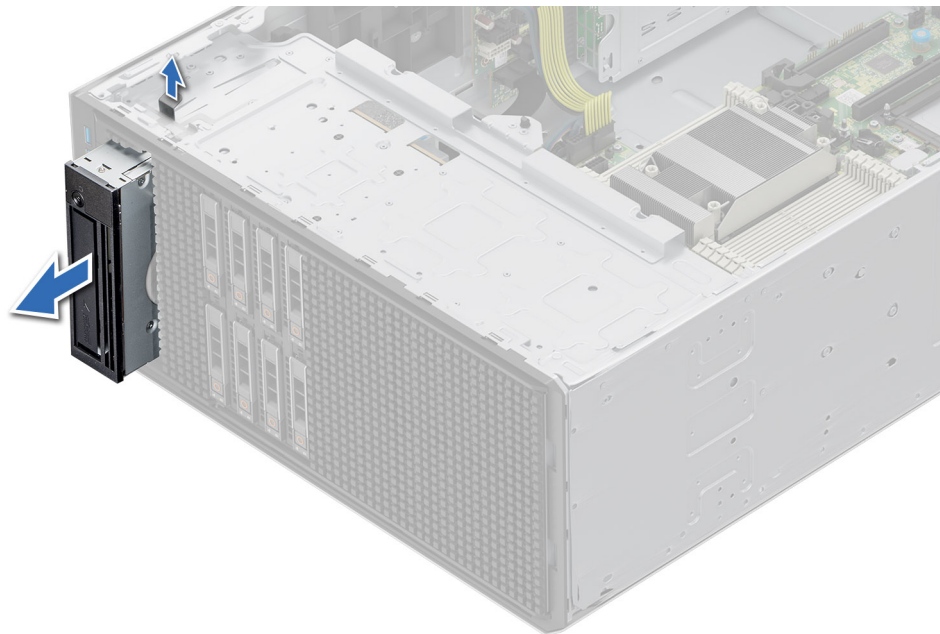
Figure 131. Retrait de l'unité de sauvegarde sur bande
