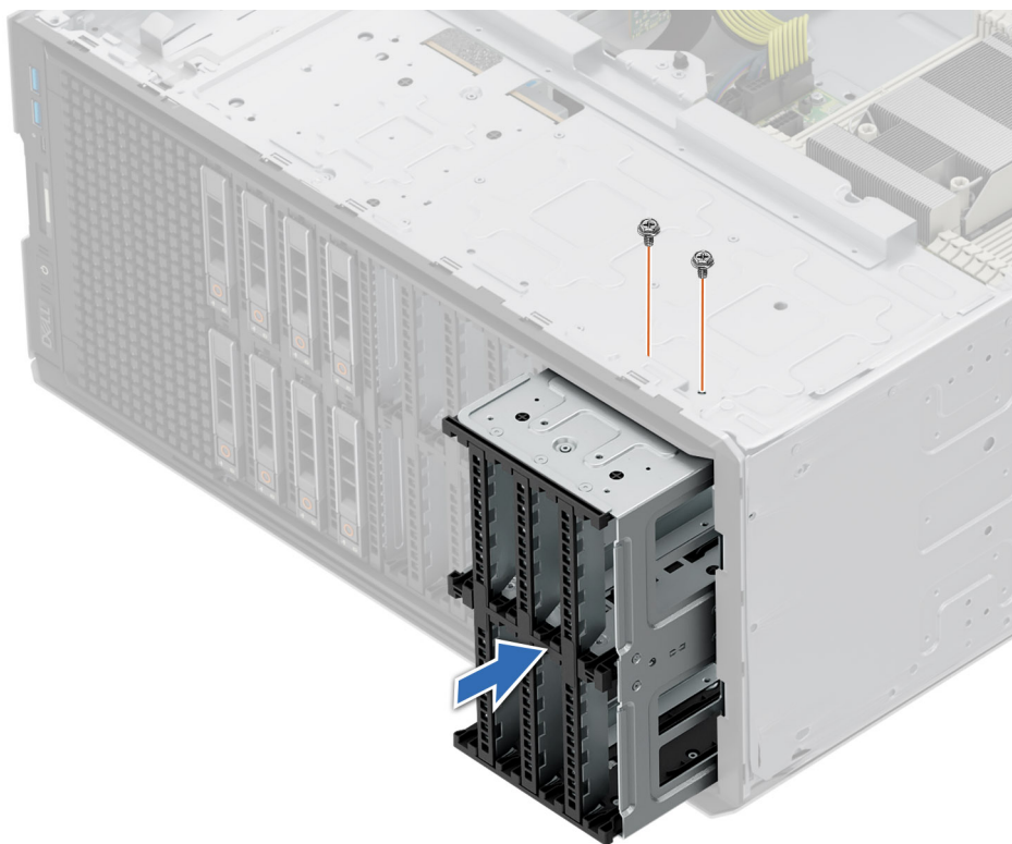
Figure 123. Installation d'une baie de disques
