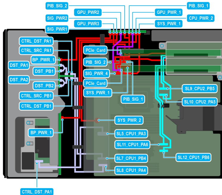
Figure 52. Configuration 14 : 8 disques de 3,5 pouces (SAS/SATA) + 8 disques de 2,5 pouces (NVMe RAID fPERC12) + 2 processeurs graphiques sur le processeur 2
