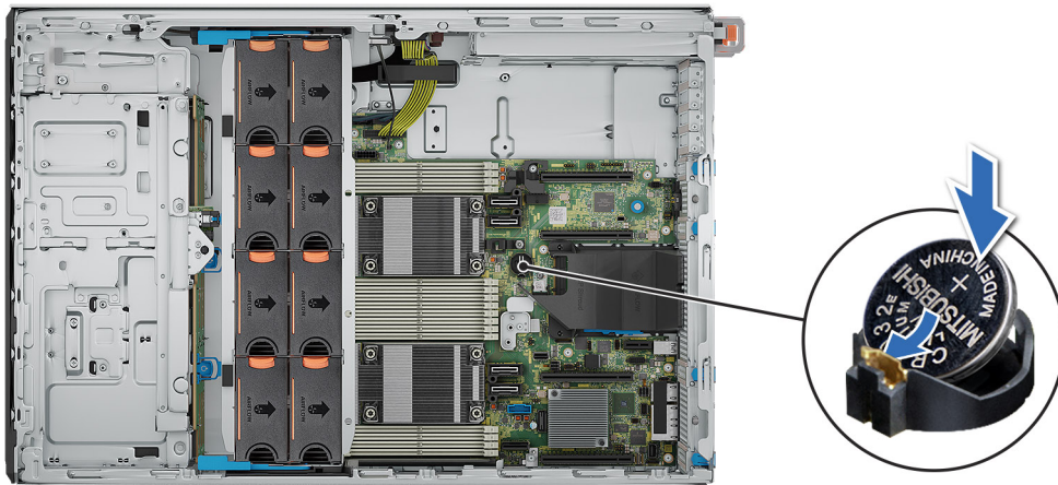
Figure 181. Installation de la pile du système
