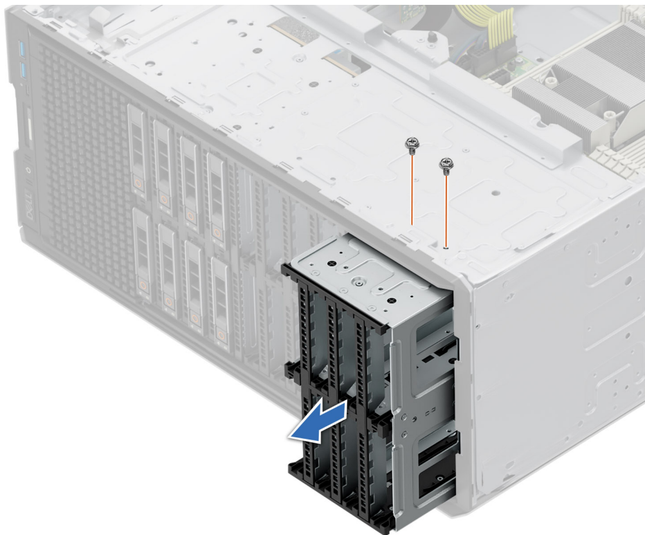
Figure 120. Retrait d'une baie de disques
