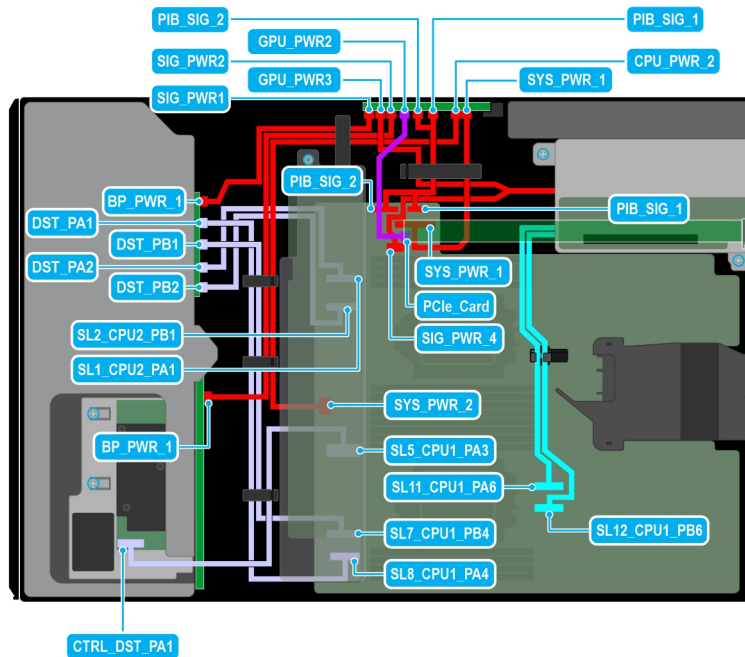
Figure 61. Configuration 23 : 8 disques de 3,5 pouces (SAS/SATA) + 8 disques de 2,5 pouces (NVMe) + 1 processeur graphique sur le processeur 2
