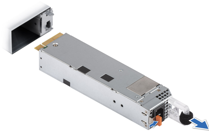
Figure 188. Retrait d'un bloc d'alimentation 60 mm
