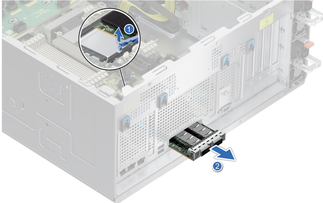
Figure 173. Retrait de la carte OCP
