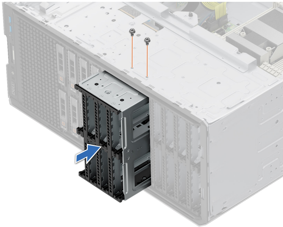
Figure 122. Installation d'une baie de disques
