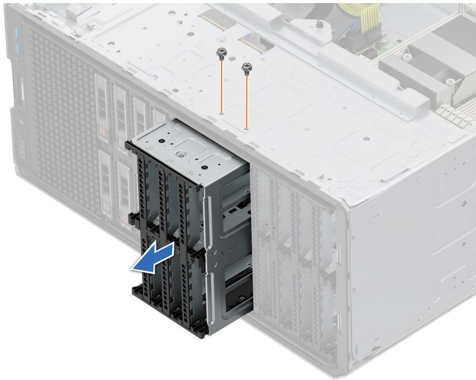
Figure 119. Retrait d'une baie de disques
