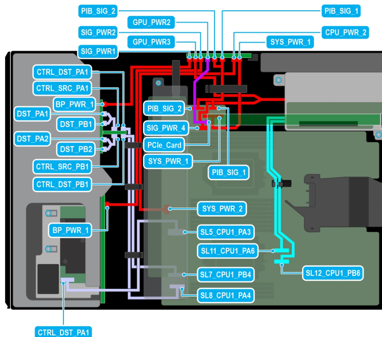
Figure 58. Configuration 20 : 8 disques de 3,5 pouces (SAS/SATA) + 8 disques de 2,5 pouces (NVMe RAID fPERC12) + 1 processeur graphique sur le processeur 2
