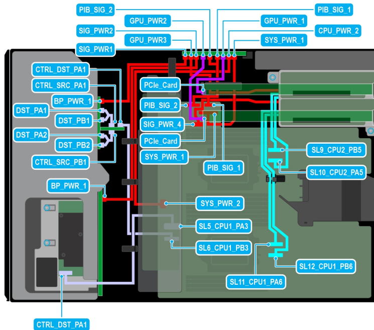
Figure 50. Configuration 12 : 8 disques de 3,5 pouces (SAS/SATA) + 8 disques de 2,5 pouces (NVMe RAID fPERC11) + 2 processeurs graphiques sur le processeur 2
