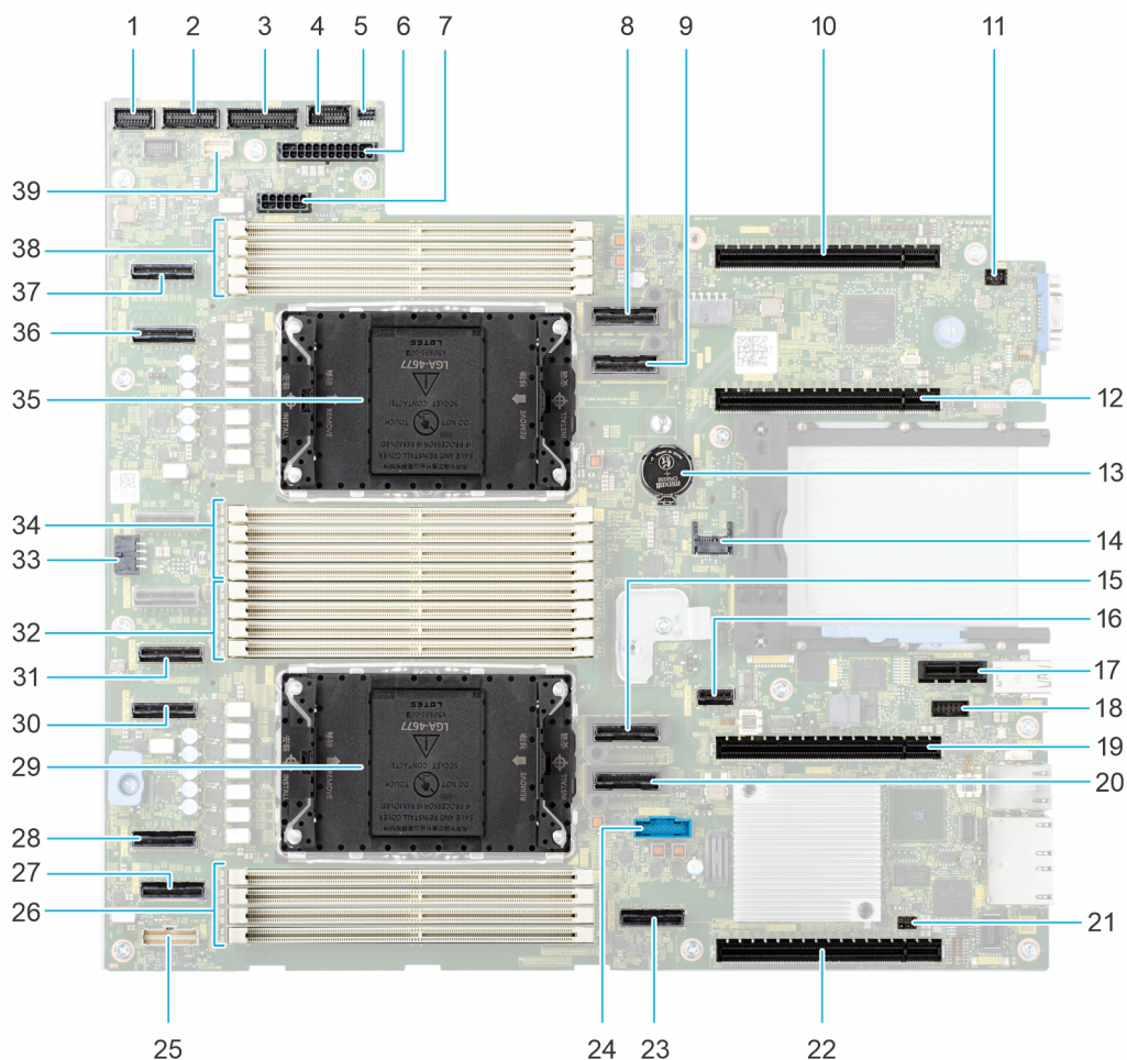
Figure 200. Connecteurs et cavaliers de la carte système
