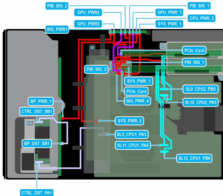
Figure 63. Configuration 25 : 12 disques de 3,5 pouces (SAS/SATA) + 2 processeurs graphiques sur le processeur 2
