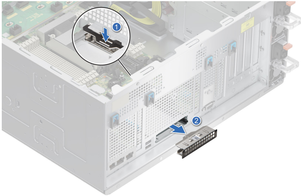
Figure 175. Retrait du cache de carte OCP
