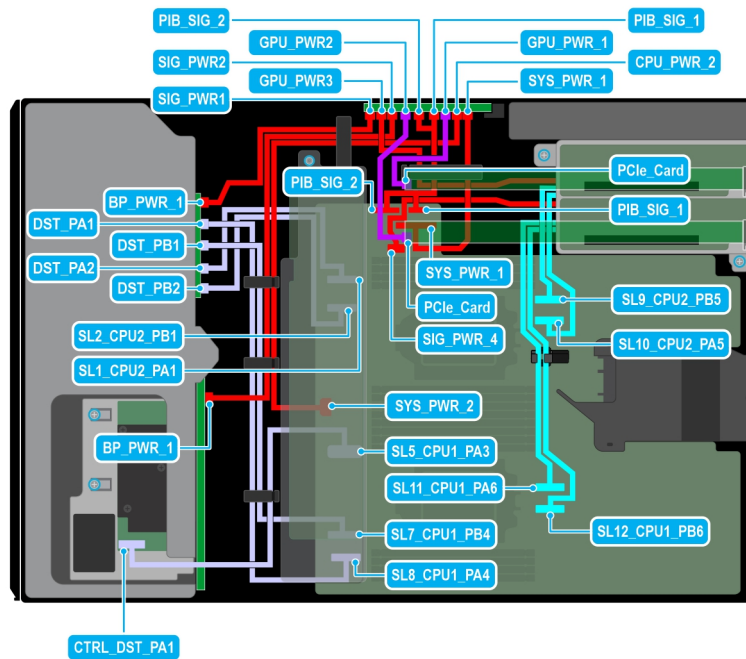
Figure 60. Configuration 22 : 8 disques de 3,5 pouces (SAS/SATA) + 8 disques de 2,5 pouces (NVMe) + 2 processeurs graphiques sur le processeur 2
