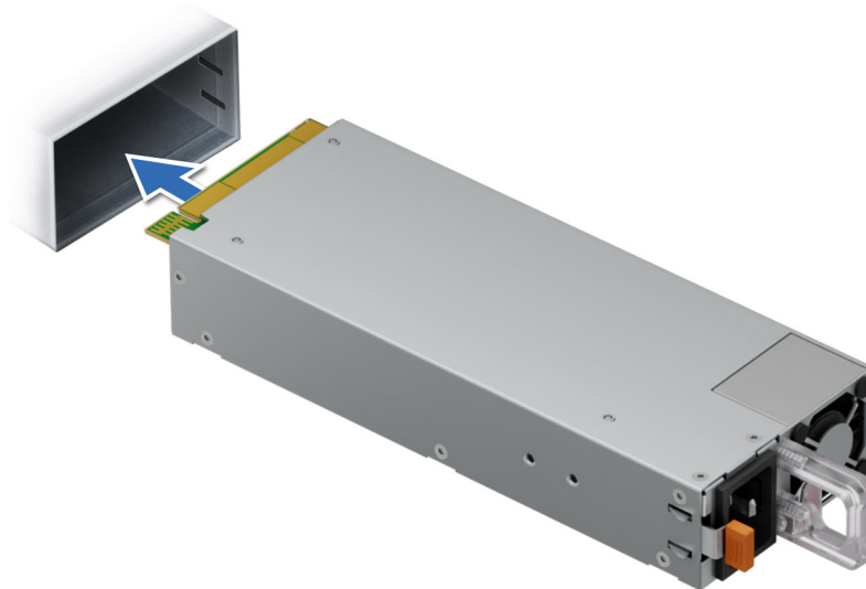
Figure 191. Installation d'un bloc d'alimentation de 86 mm
